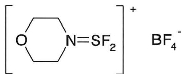
XtalFluor-M +
