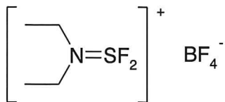
XtalFluor-E +
